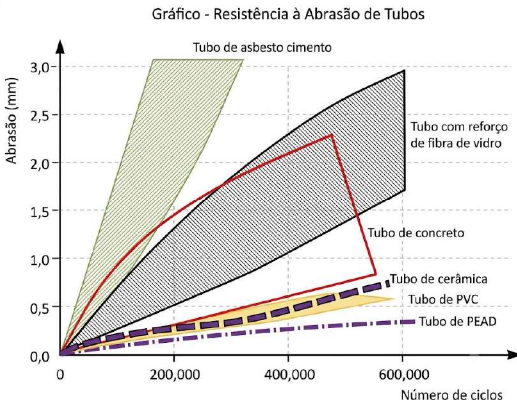
Figura 3 - Gráfico de Abrasão (DIN 19534) - Universidade de Darmstadt
