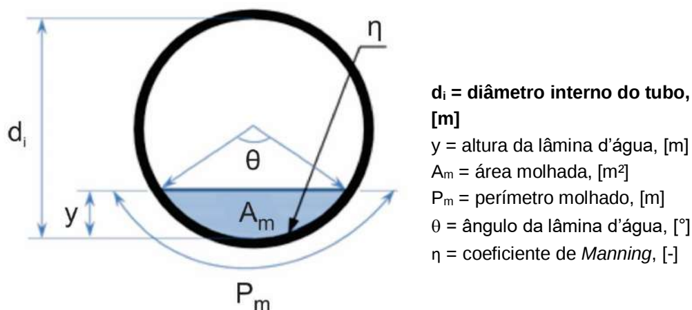
Figura 33 - Variáveis para dimensionamento hidráulico
