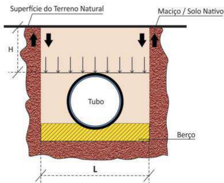
Figura 30 - Carga de solo atuante
