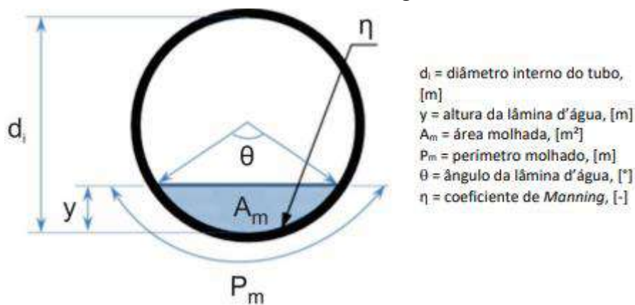
Figura 33 - Variáveis para dimensionamento hidráulico
