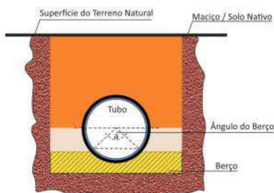
Figura 32 – Ângulo do berço
