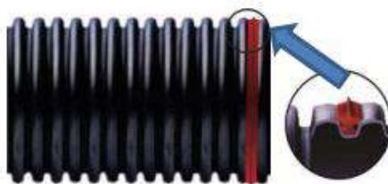
Figura 37 - Detalhe do anel de vedação instalado
