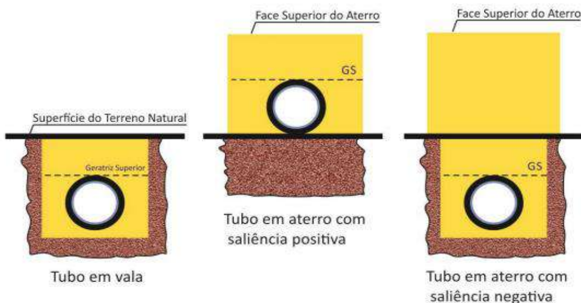
Figura 24 - Condições de Instalação de tubos em vala ou aterro
