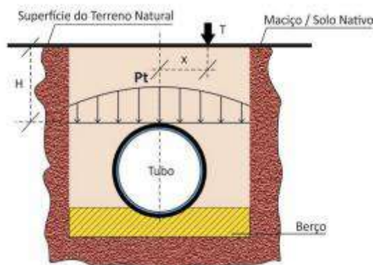
Figura 31 - Carga de tráfego
