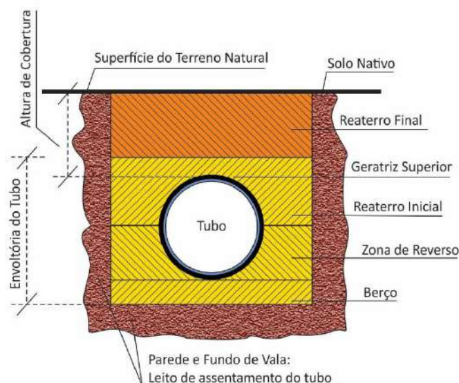
Figura 28 – Tubo enterrado – definição das partes integrantes de uma instalação típica
