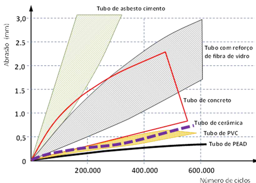
Figura 3 - Gráfico de Abrasão (DIN 19534) - Universidade de Darmstadt
