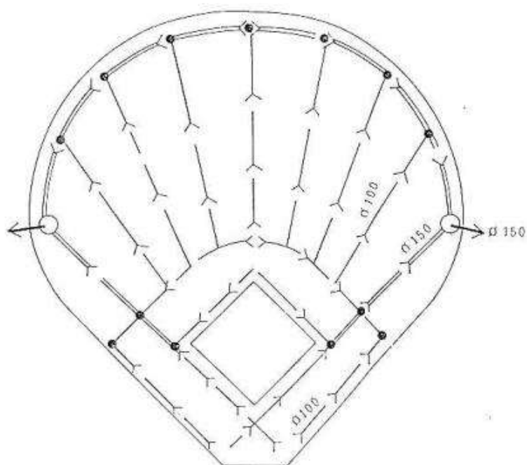
Figura 26- Exemplo de sistema drenante em campos de Baseball
