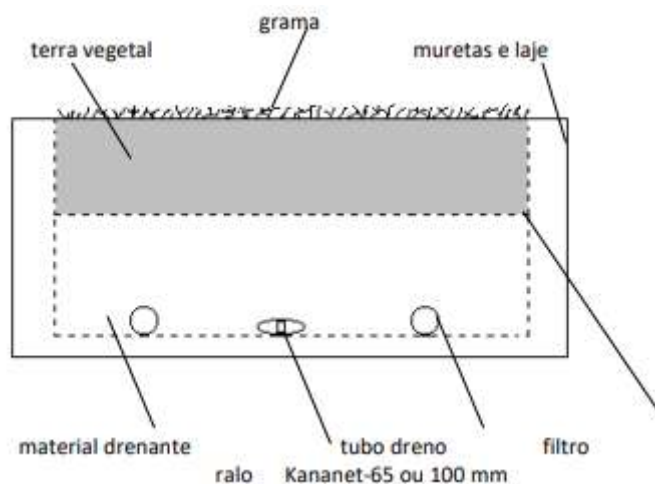
Figura 19 – Seção esquemática de colchão drenante sobre laje, a colocação dos tubos drenos Kanaflex permite uma captação mais rápida das águas, diminuição na altura necessária do colchão drenante e maior espaçamento entre ralos.
