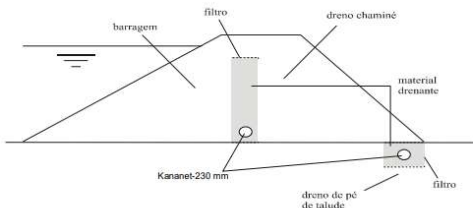
Figura 21 – Seção transversal de barragem de terra, dotada de dreno chaminé para interceptar as águas infiltradas pelo talude de montante e de dreno de pé de talude para interceptar o fluxo pelas fundações.
