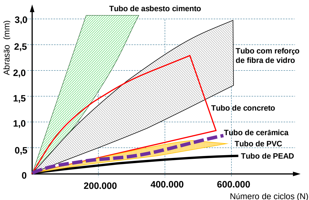
Gráfico - Resistência à Abrasão de Tubos
